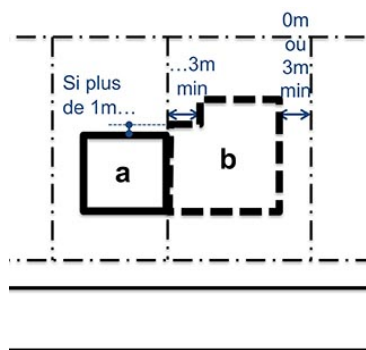
Recul latéral des constructions principales*
