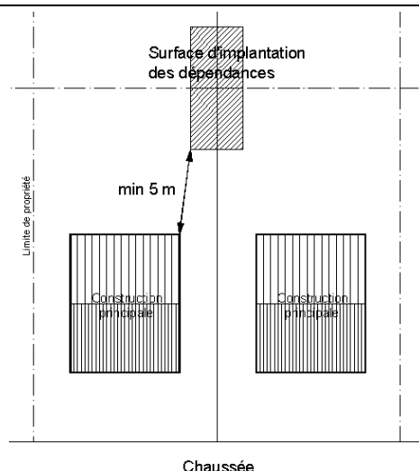
Reculs des dépendances
