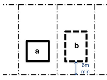
Recul avant des constructions principales*
