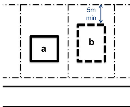
Recul arrière des constructions principales*
